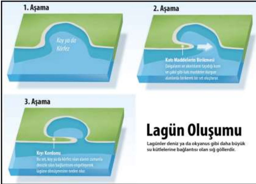
Şekil 1. Lagün oluşumu ( https://bilimgenc.tubitak.gov.tr/makale/deniz-kiyisindaki-goller-lagunler )
