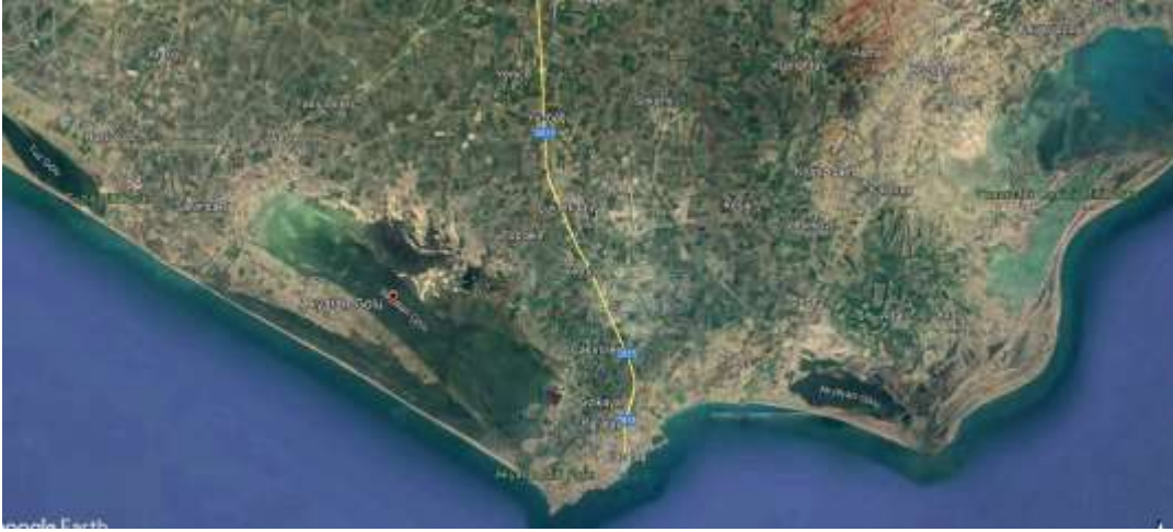
Şekil 2. Tuz Gölü, Akyatan, Ağyatan ve Yumurtalık lagünleri(google earth 2024).
